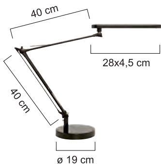
Interruttore ON/OFF sotto la calotta
